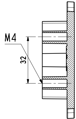
Sez. A-A
